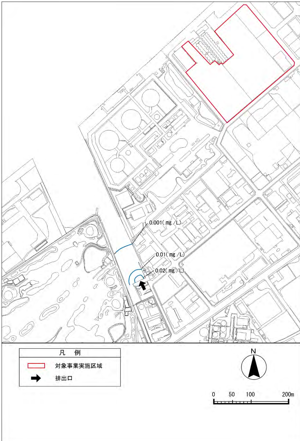
図 6.5.3(1) 水の汚れ（化学的酸素要求量）の予測結果（寄与濃度）
