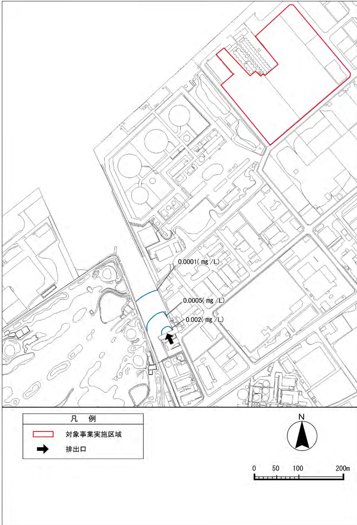
図 6.5.3(3) 水の汚れ（全磷）の予測結果（寄与濃度）
