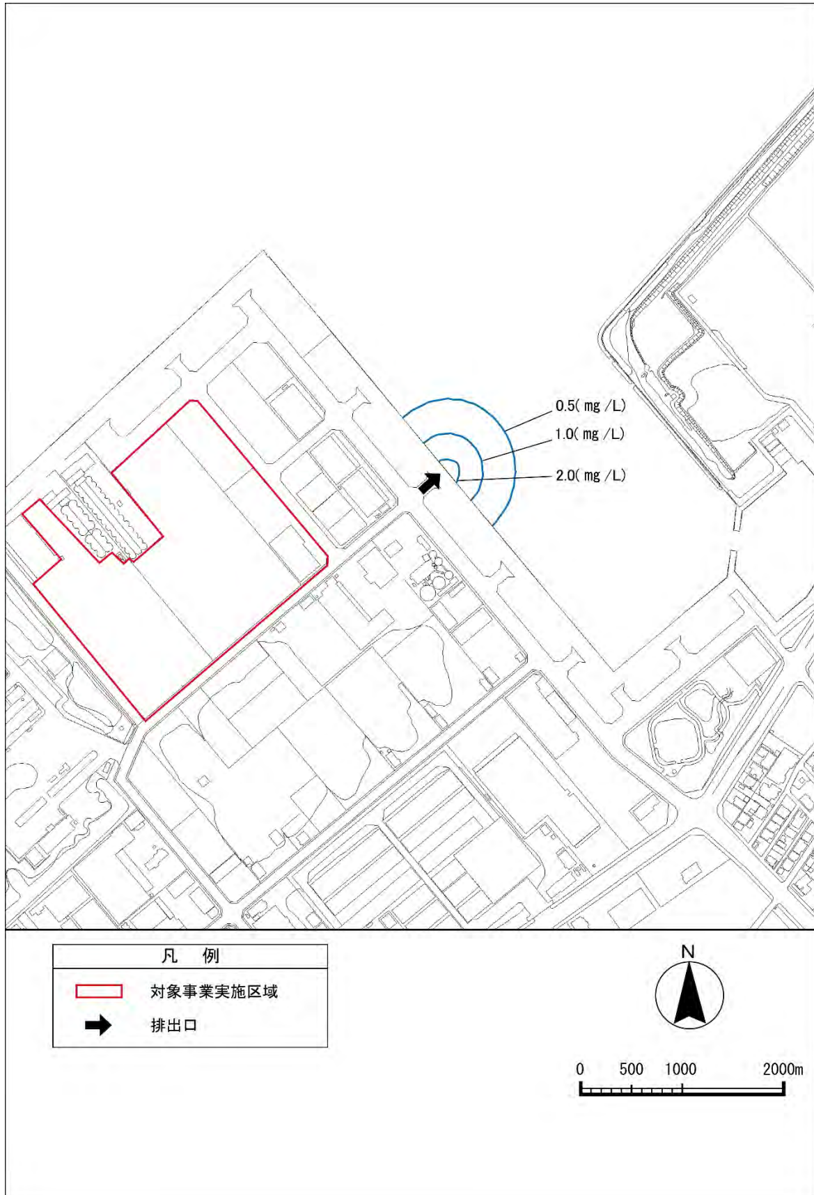
図 6.5.2 水の濁り（浮遊物質濃度）の予測結果（寄与濃度）
