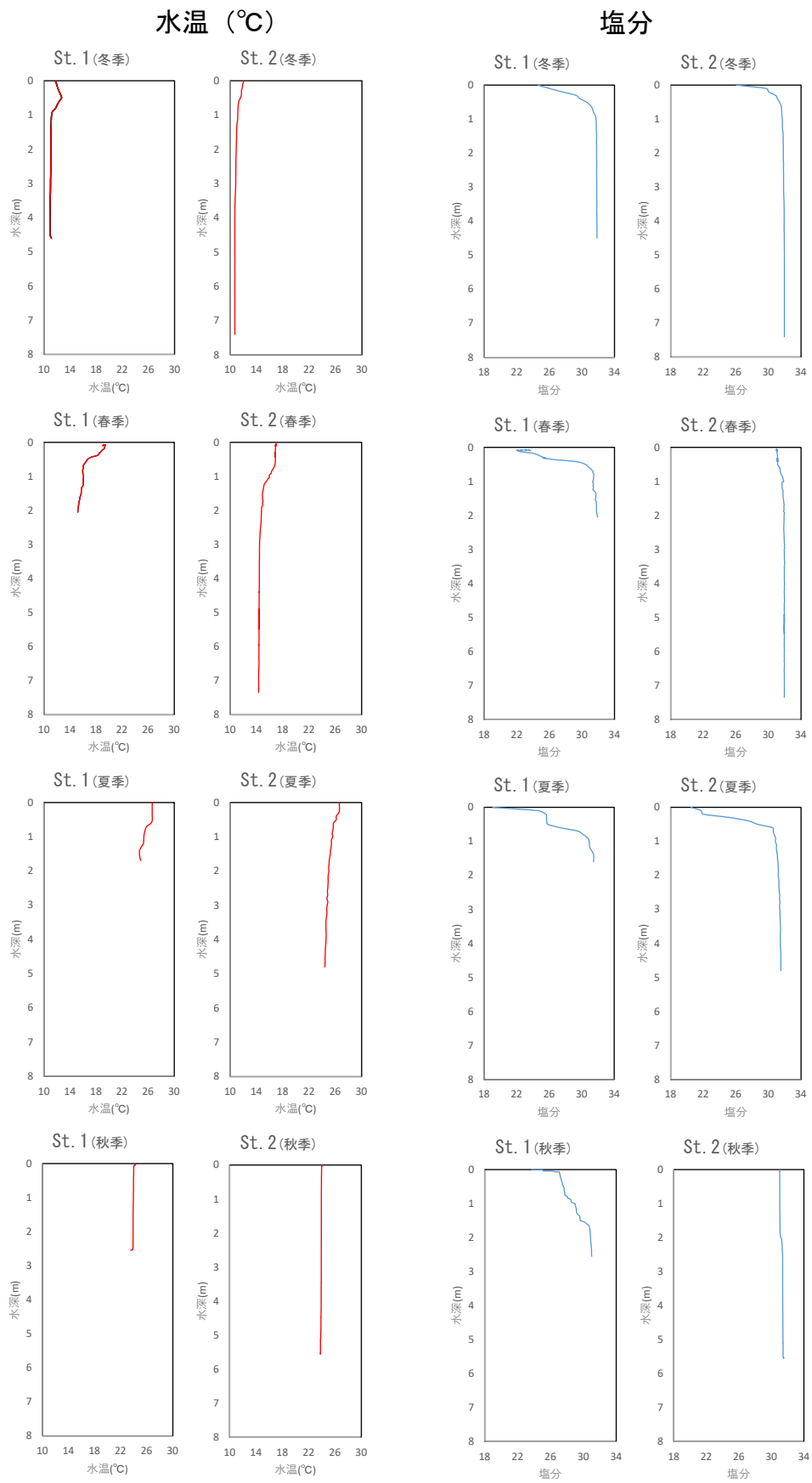
図 6.5.4 水温・塩分鉛直分布（季節別）
