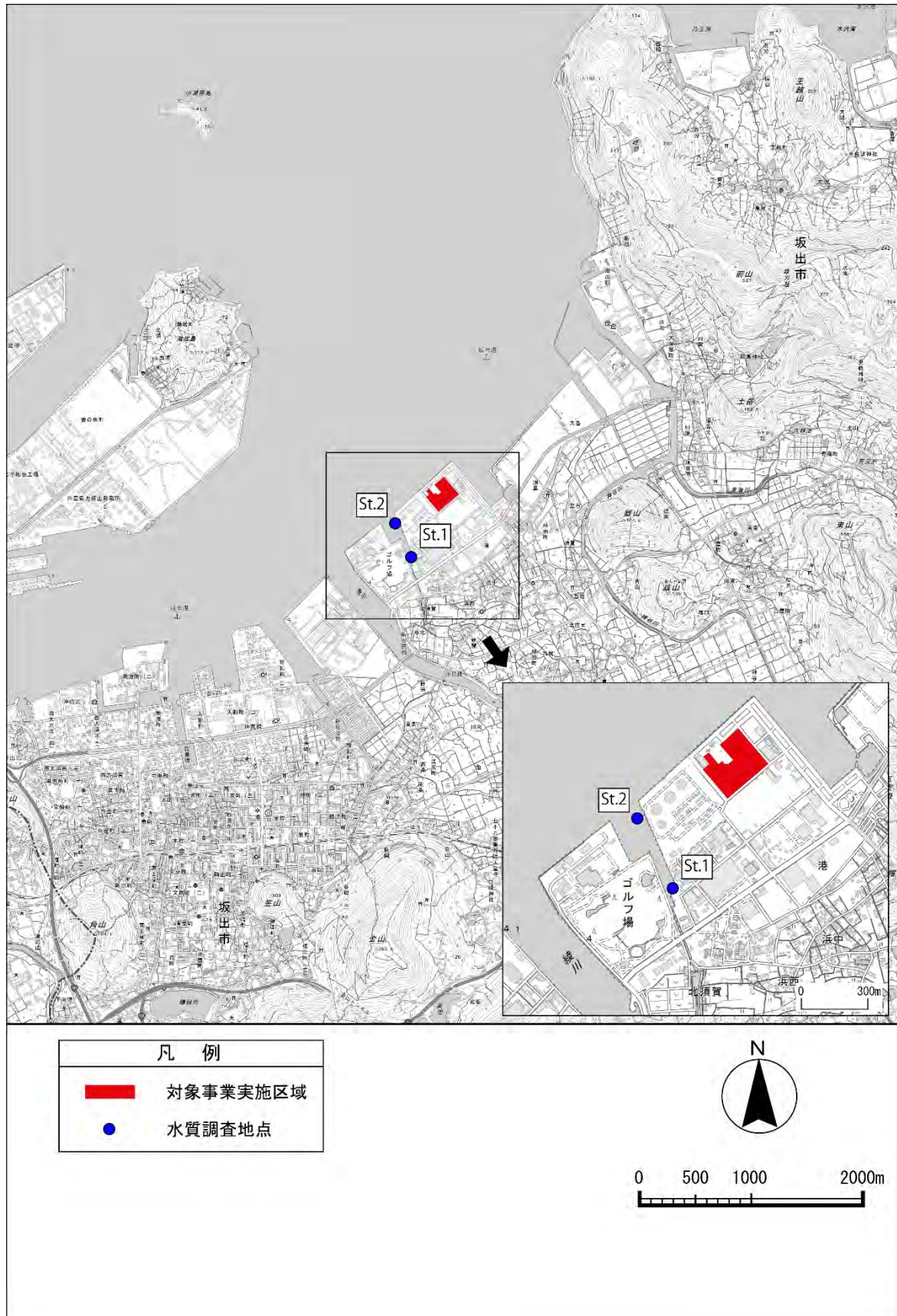
図 6.5.1 水環境調査位置（水質）
