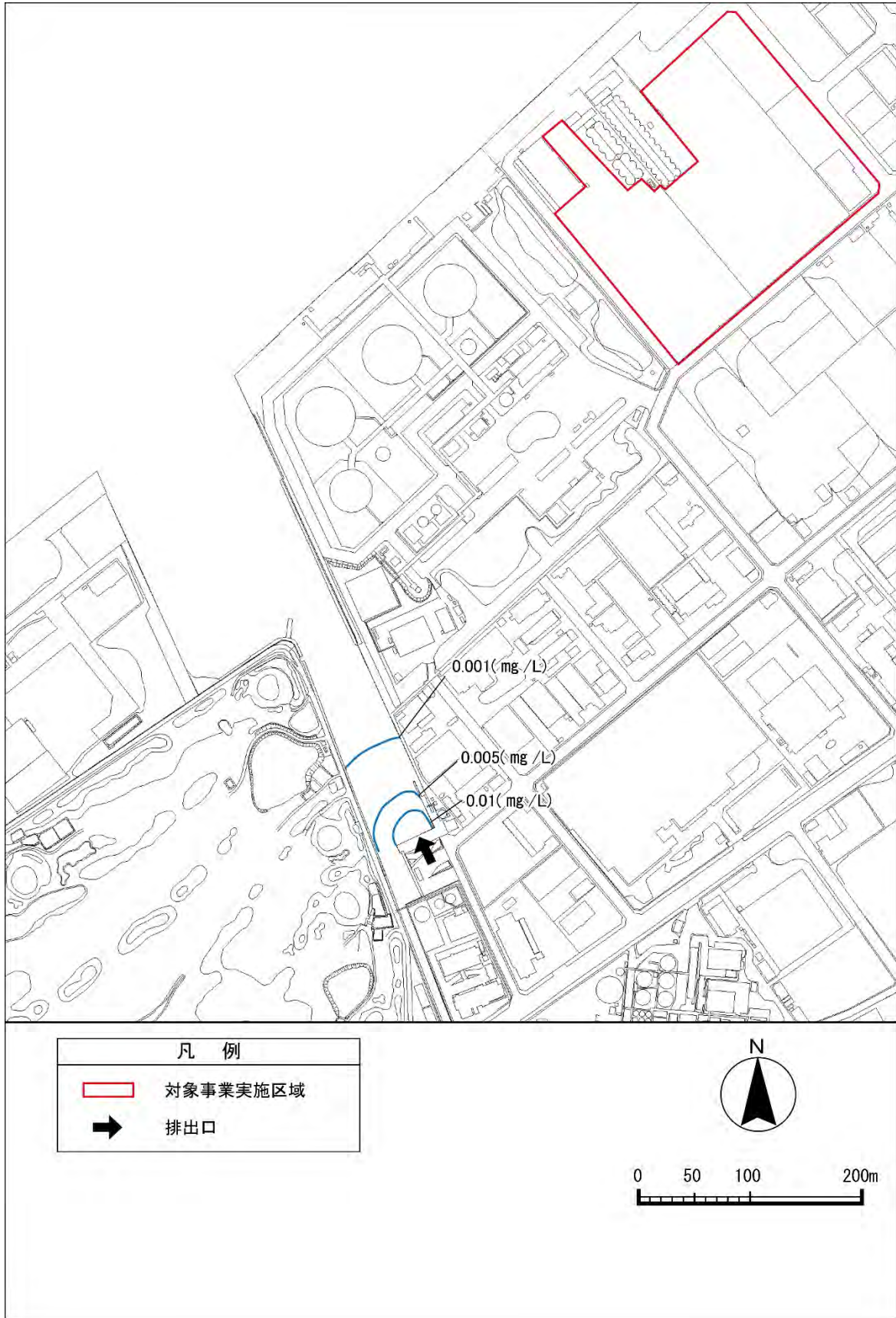
図 6.5.3(2) 水の汚れ（全窒素）の予測結果（寄与濃度）
